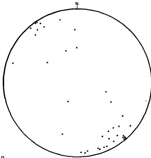
FIGURA N° 4.- Proyección equiareal de la lineación L (58) en la Formación Limolitas del Pusa (Arroyo de Fuentes, Río Huso y corte del F.C.)
