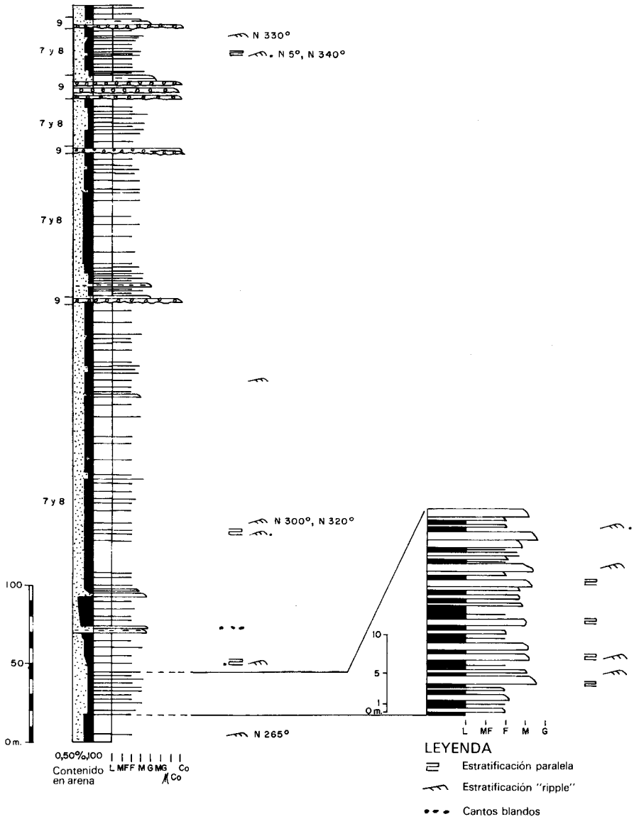
FIG. 1.-COLUMNA SEDIMENTOLÓGICA DE LA ESTRELLA (F. ESTOMIZA)
