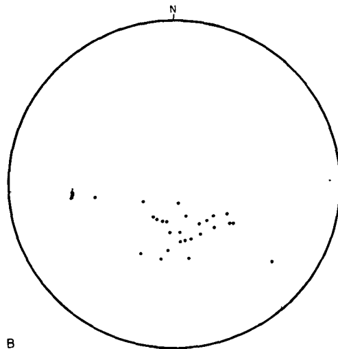
Figura N° 6 A.- Proyección equiareal de los polos (22) de la foliación y bandeado de las migmatitas y anatectitas de Azután. B.- Proyección equiareal de los polos (26) de la fluidalidad planar del granito de Aldeanueva de Barbarroja.
